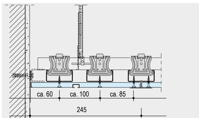
Schnitt D-D
